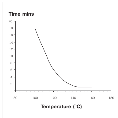
Gel time
